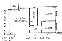
PIANO PRIMO
